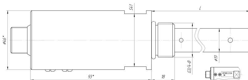
Рис.2 Габаритный чертеж датчика ВТИЮ.3124-03
