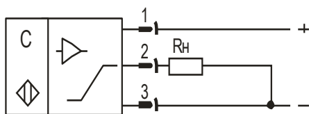
Рис.3 Схема подключения датчика ВТИЮ.3124-03
