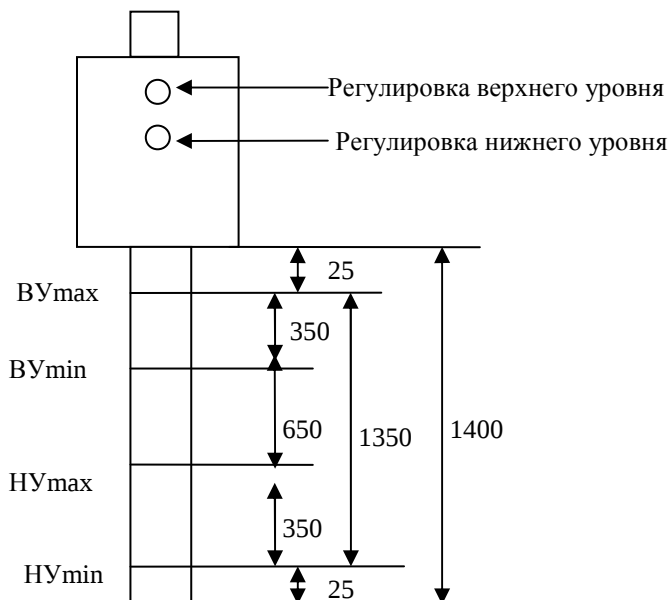
Рис.1 Датчик уровня ВТИЮ.3124-03
